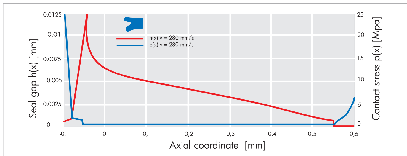
Bild 02: Kontaktspannung p und Kontakthöhe h Nutring T20
