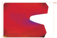
Merkel Nutring T20 bei 20 MPa
