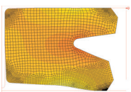
Merkel Nutring T20 bei 0 MPa
