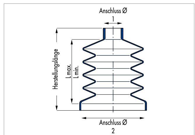
Maßskizze Mehrfaltenbalg
