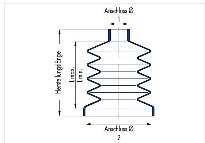
Maßskizze Mehrfaltbalg
